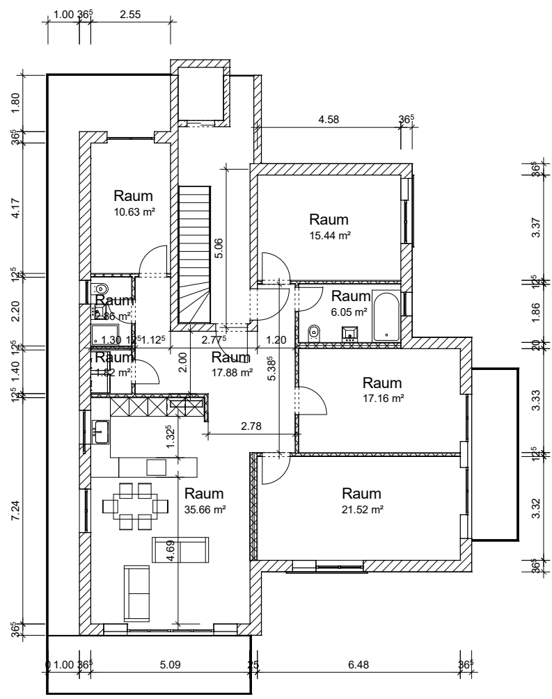
Dachgeschoss
