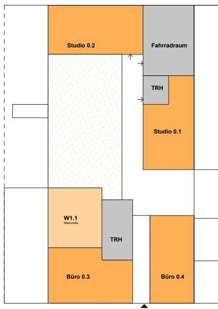
Lageplan EG
