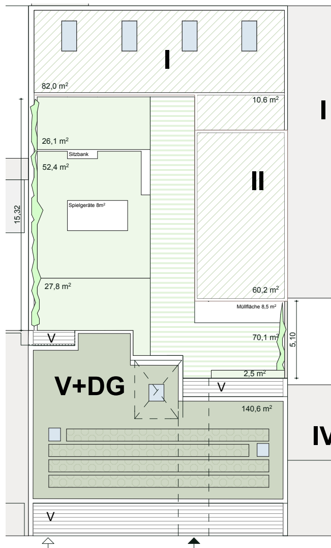
Lageplan | Dachaufsicht
