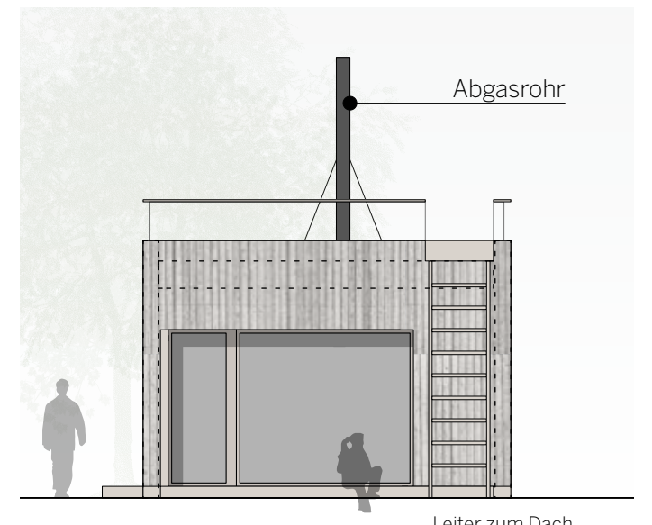
ANSICHT NORD-OST
