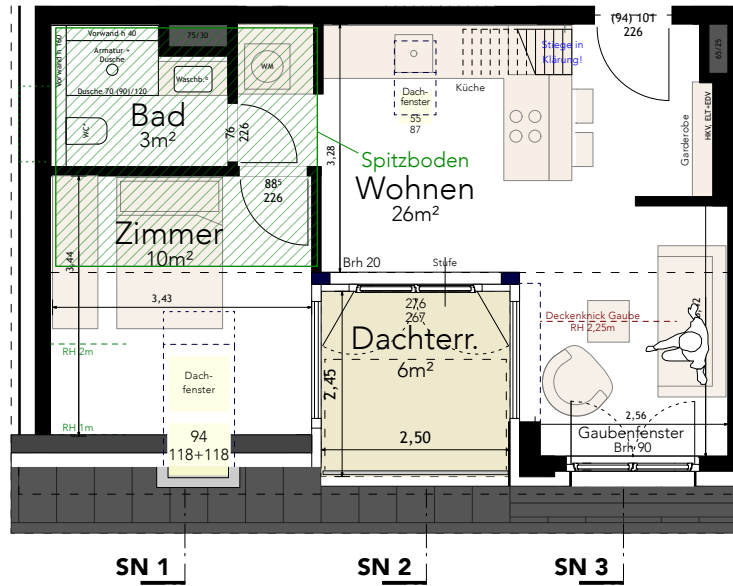
GRUNDRISS WOHNEBENE
