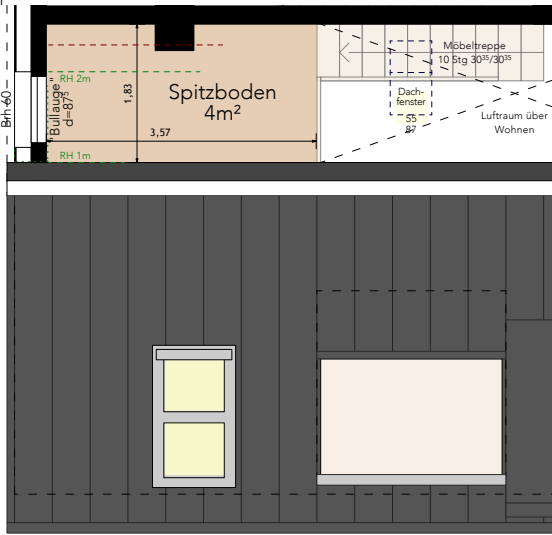
GRUNDRISS SPITZBODEN
