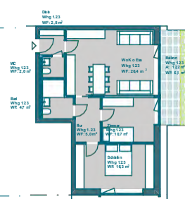
Variante 3-Zimmer-Wohnung mit zusätzlichem WC
