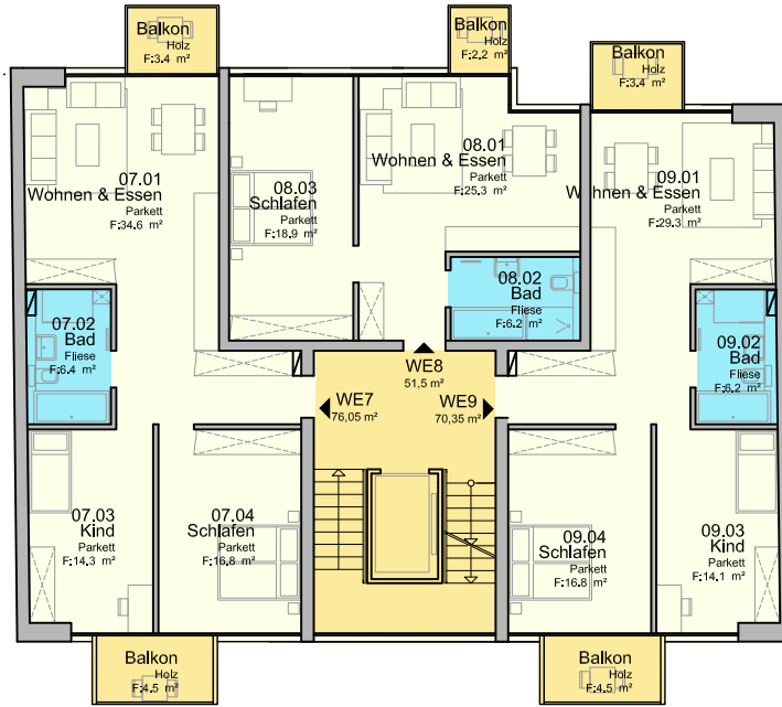
Grundriss 2. Obergeschoss
